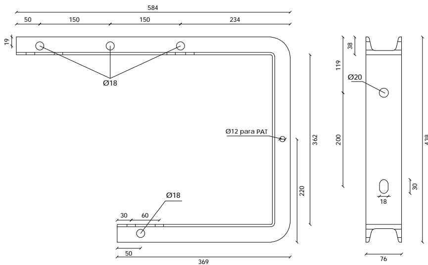
ALZADO
